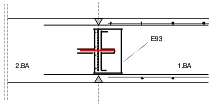
Arbeitsfuge bei Aussenwand
